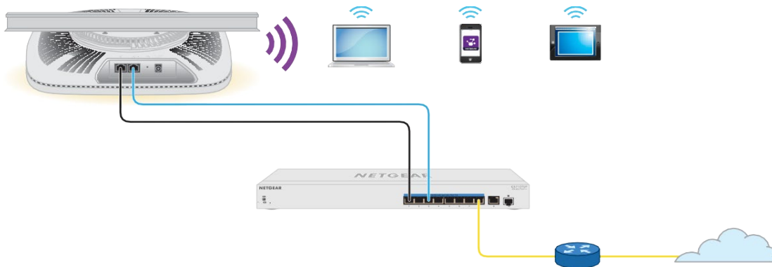
図9.リンクアグリゲーション接続
