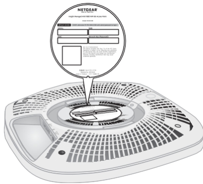
図3.アクセスポイントラベルの位置
