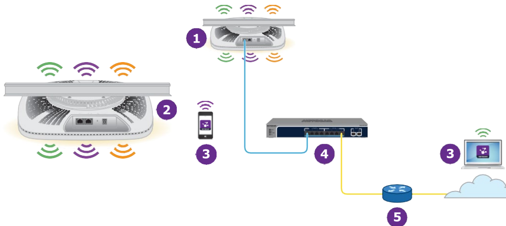
図8. ノードを有線ルートに接続する
